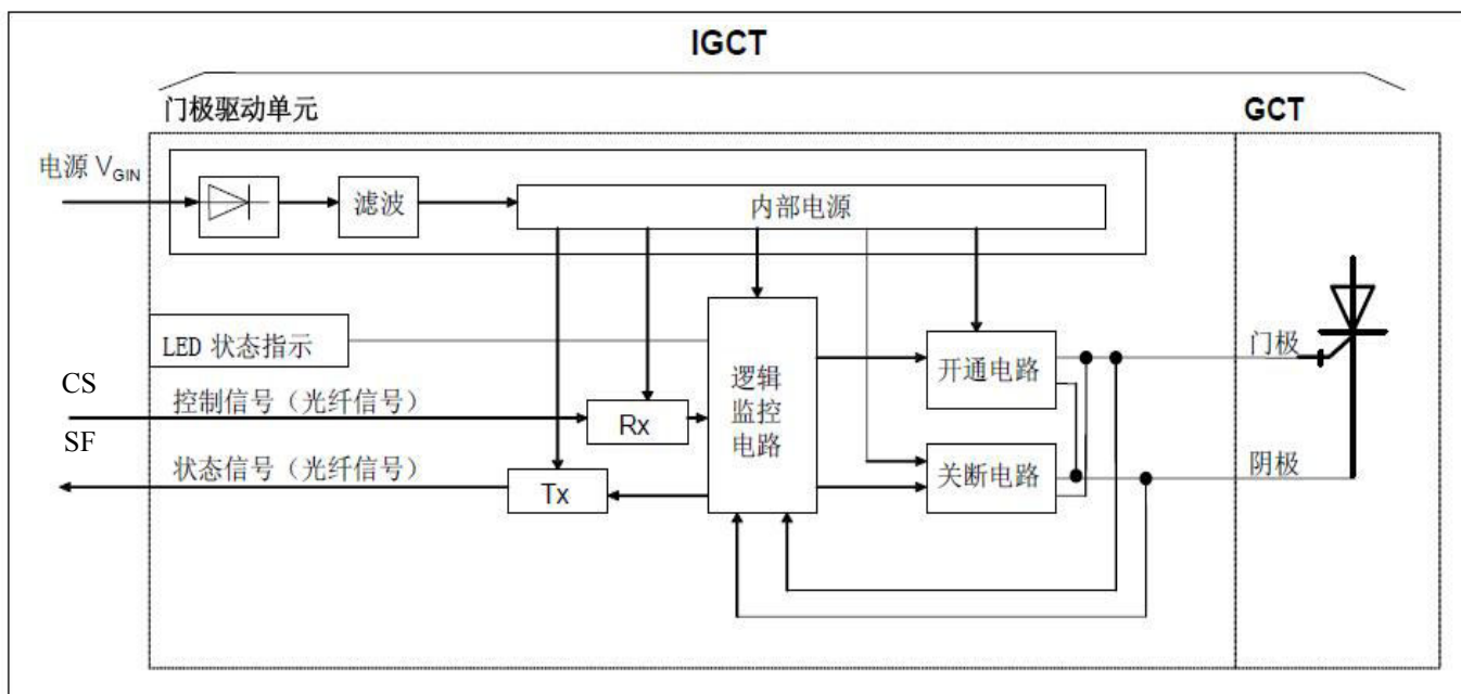
图10. IGCT器件门极电路框图
