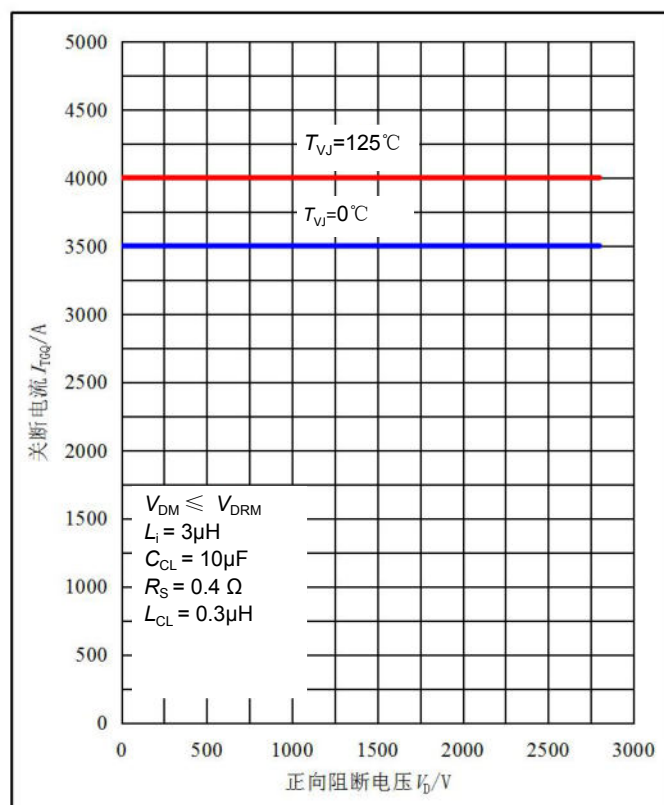
图3. 安全工作区
